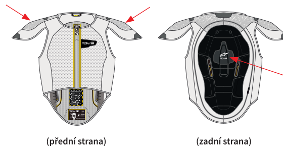
obrázek 1 – umístění senzorů
